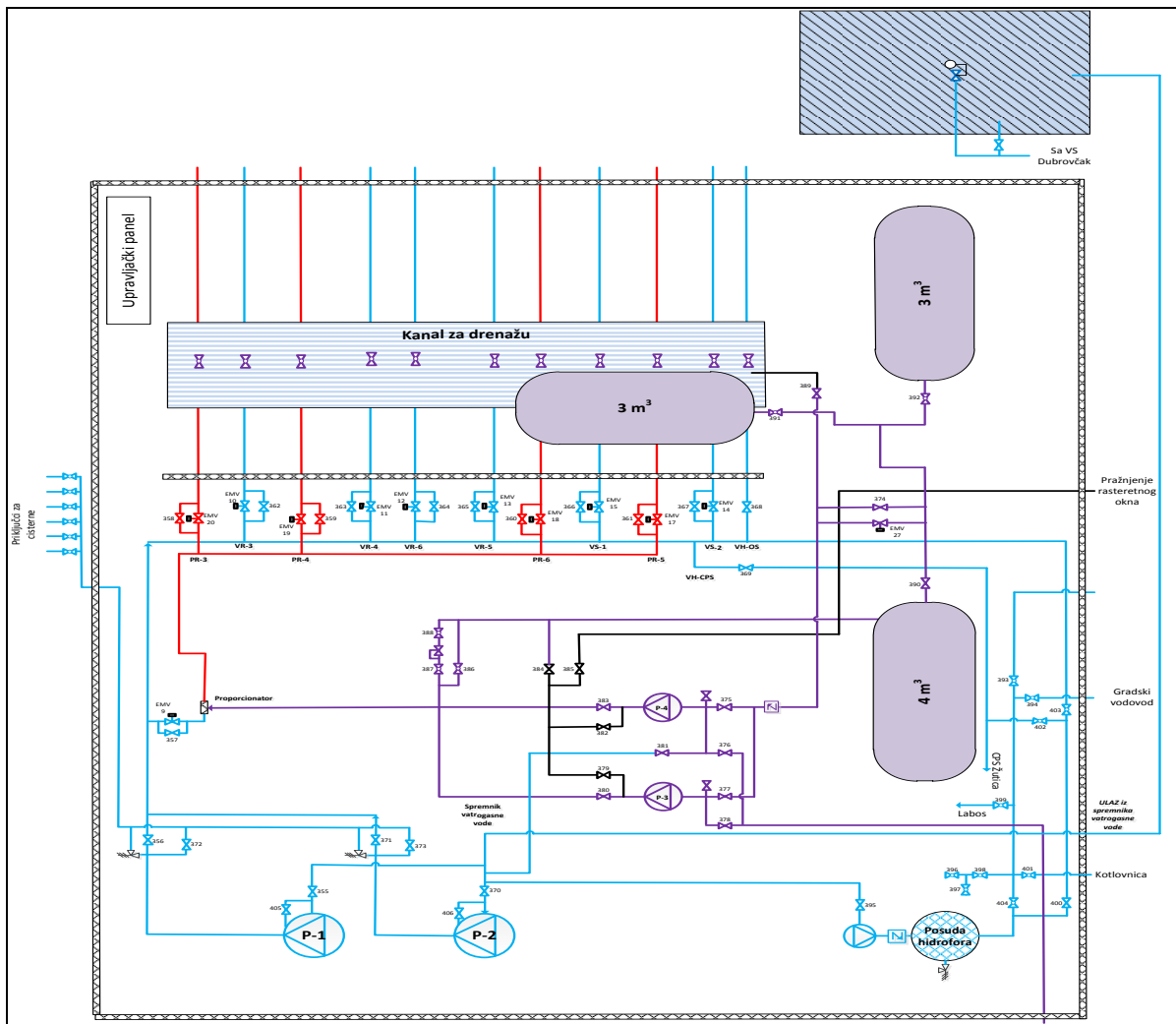
Slika 40. Shema vatrogasnice [2]
