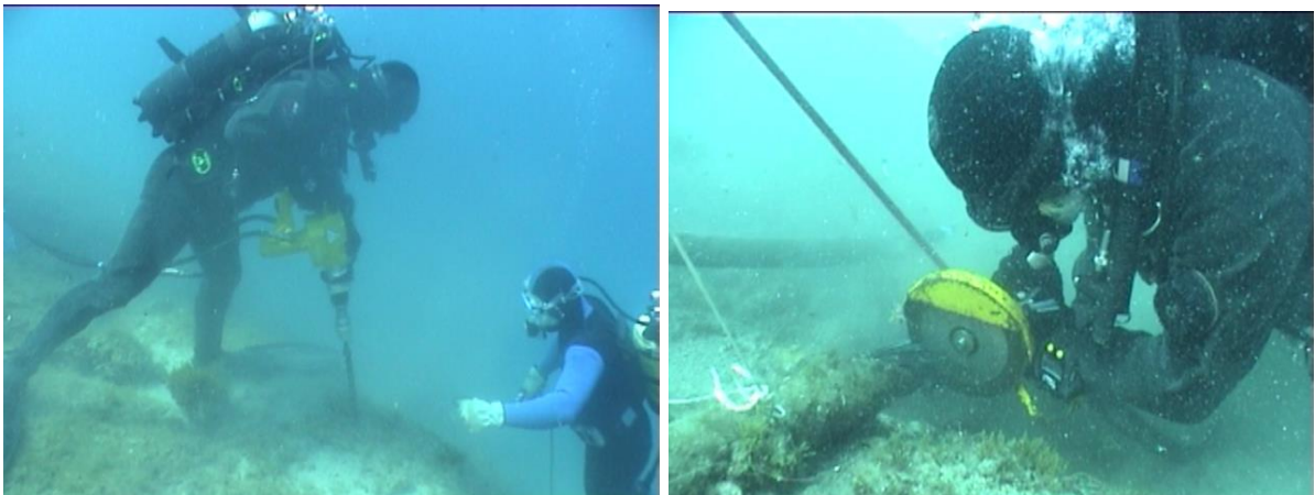
SLIKE 3 i 4.radovi sa hidrauličkom bušilicom i hidrauličkom brusilicom
