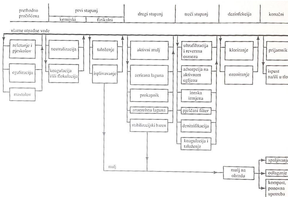
Slika 4. Dijelovi tehnološke linije pročišćavanja otpadnih voda [4]
