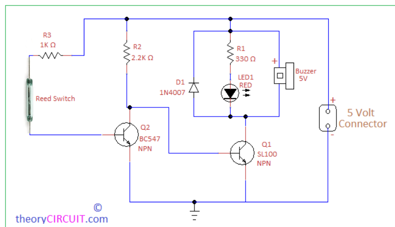
Slika 22. Shema alarmnog sustava sa reed senzorom za vrata i prozore
