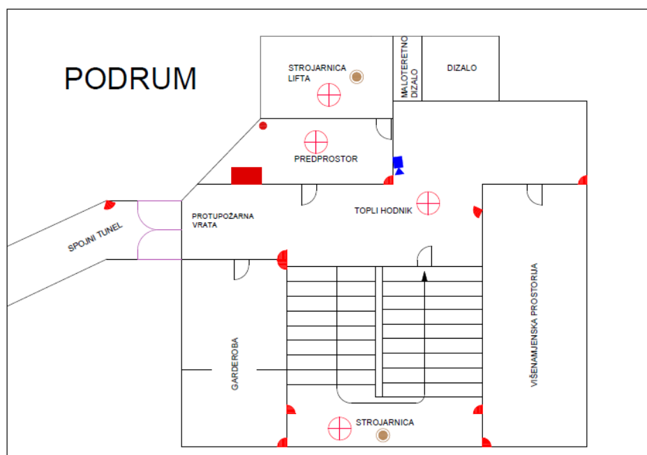
Slika 32. Skica tlocrta podruma sa rasporedom elemenata tehničke zaštite [Izvorno autor]
