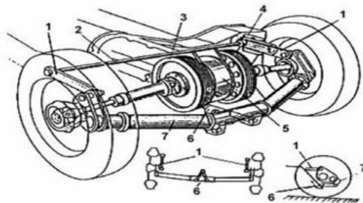
Slika 6. Mehanizam za vođenje pogonskih upravljivih kotača. [1]
