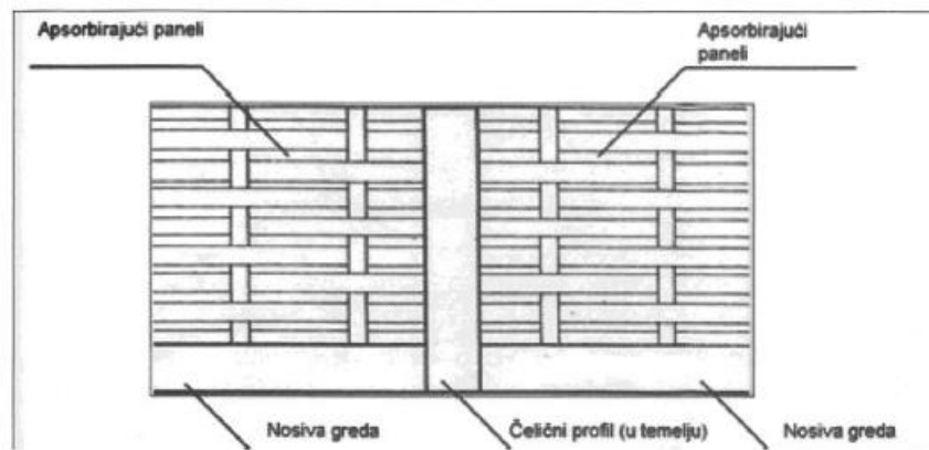
Slika 21. Elementi zidova
