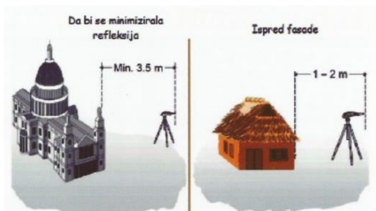
Slika 10. Položaj mikrofona van
