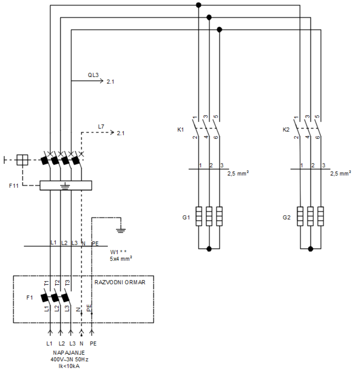
Slika 45. Energetska shema TermoBlok
