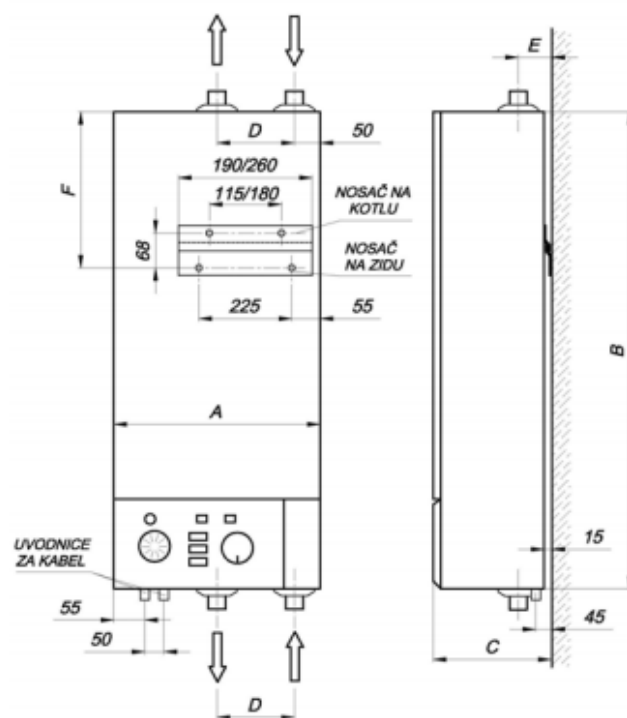
Slika 11. Dimenzije kotla [13]
