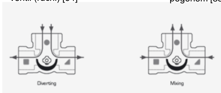
Slika 28. 3-putni miješajući ventil (ručni) [34]
