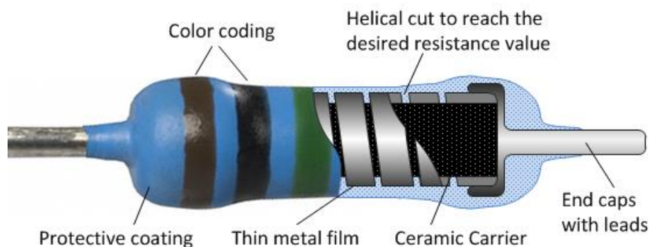
Slika 7 Struktura otpornika [8]
