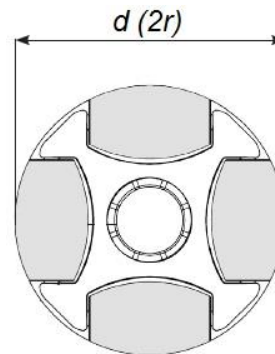
Slika 7: Dimenzije kotača.
