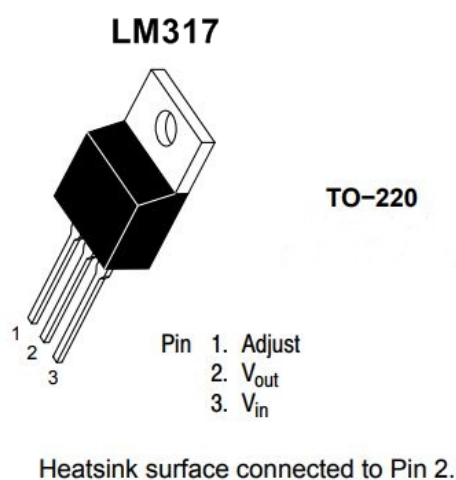
Slika 9: LM317 [15]
