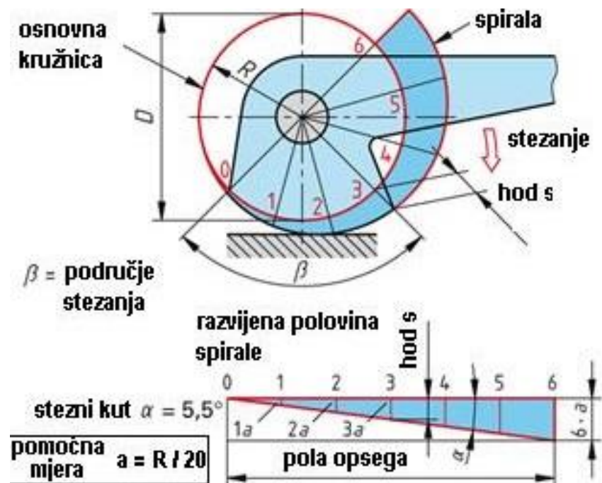
Slika 8. Spiralni ekscentar [1]
