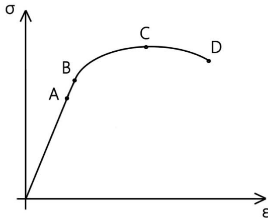
Slika 9. Graf ovisnosti deformacije o naprezanju [6]
