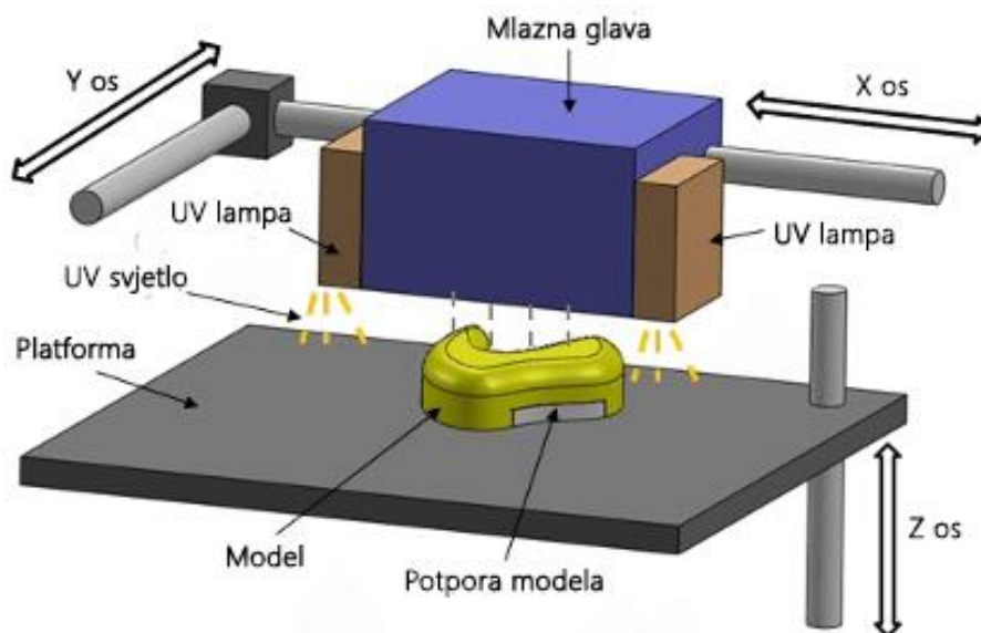
Slika 14. PolyJet tehnologija [14]
