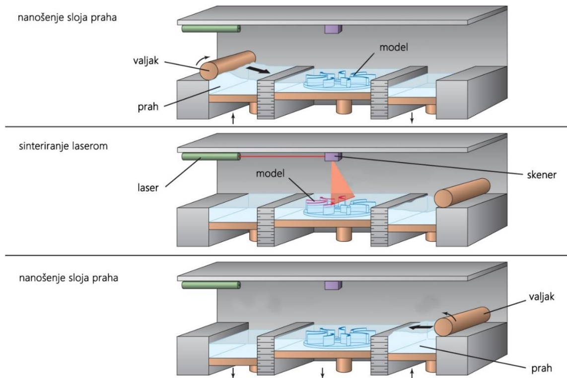
Slika 16. SLS tehnologija [16]
