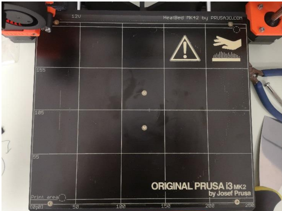
Slika 35. Grijana platforma
