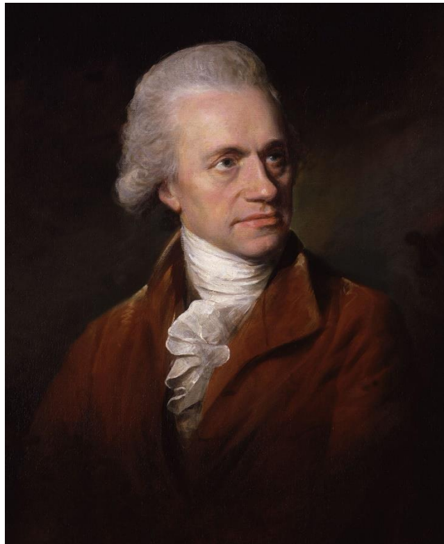
Slika 9.: William Herschel [11]
