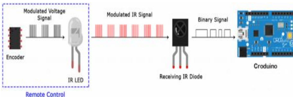
Slika 21. Prikaz infracrvene komunikacije [26]
