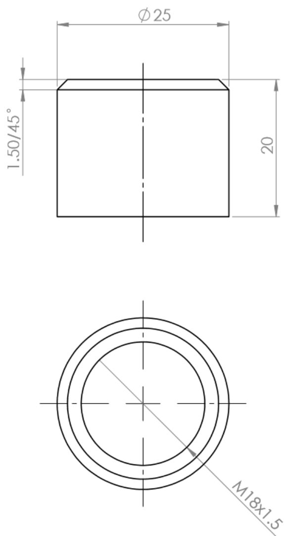
Slika 25. Priključnica nacrt.
