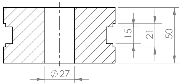
PRESJEK A-A
