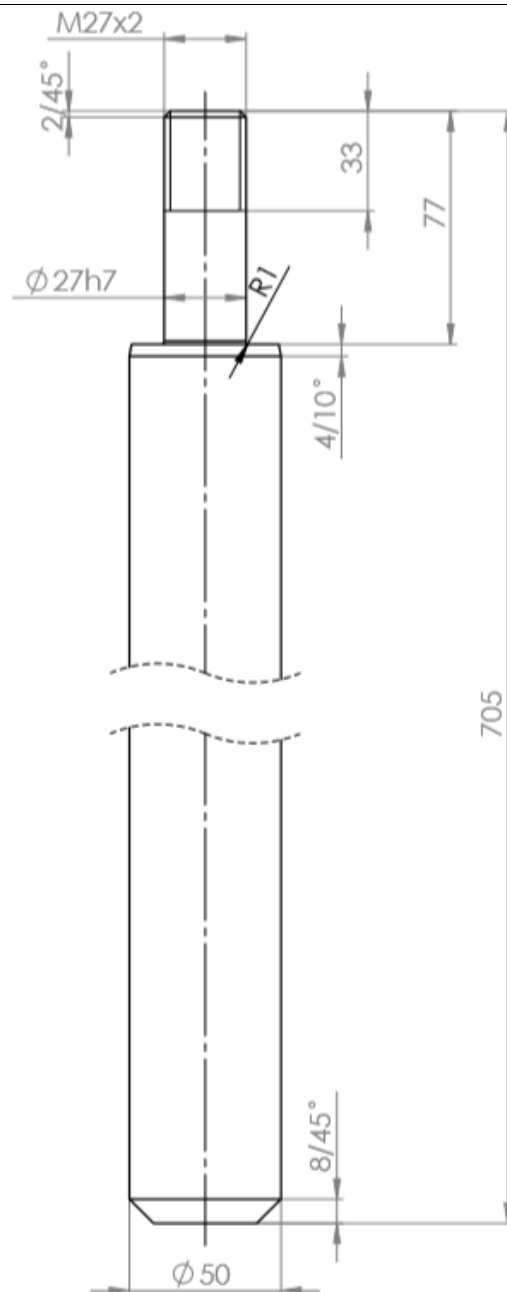
Slika 11. Klipnjača nacrt.
