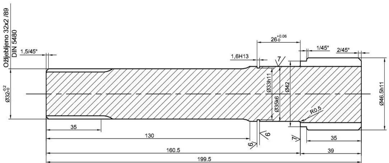
Slika 37. Crtež zupčanika redukcije
