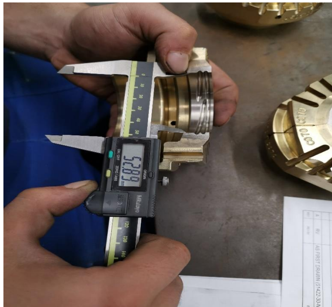
Slika 56: Kontrola promjera fazone pomičnim mikrometrom.
