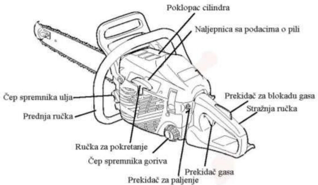
Slika 26 Dijelovi motorne pile lančanice [18]
