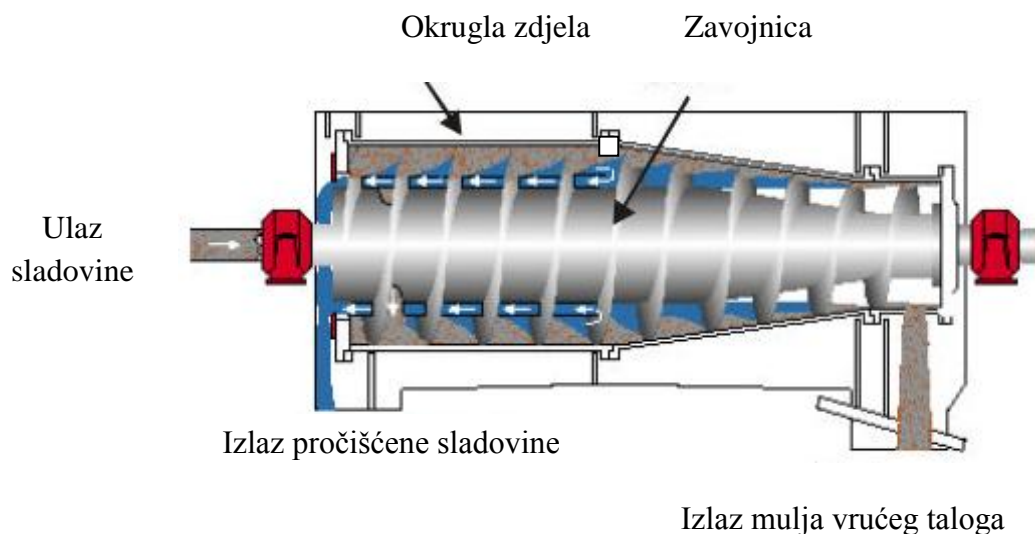
Slika 2. Shema principa rada dekanter centrifuge
