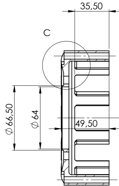
SECTION A-A
