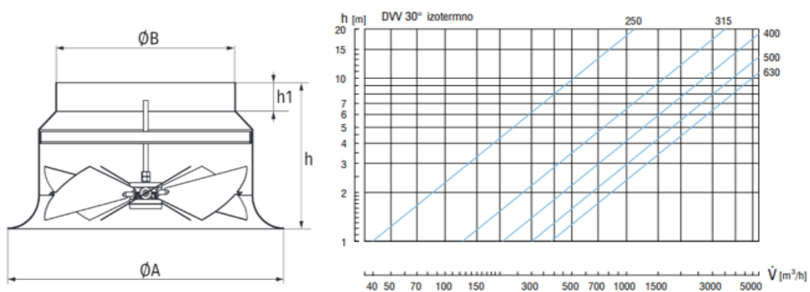
Slika 7.1. Stropni distributer DVV-500 [17]
