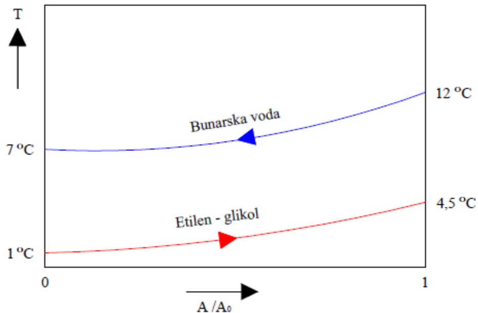
Slika 6.2. T – A dijagram međuzmjenjivača
