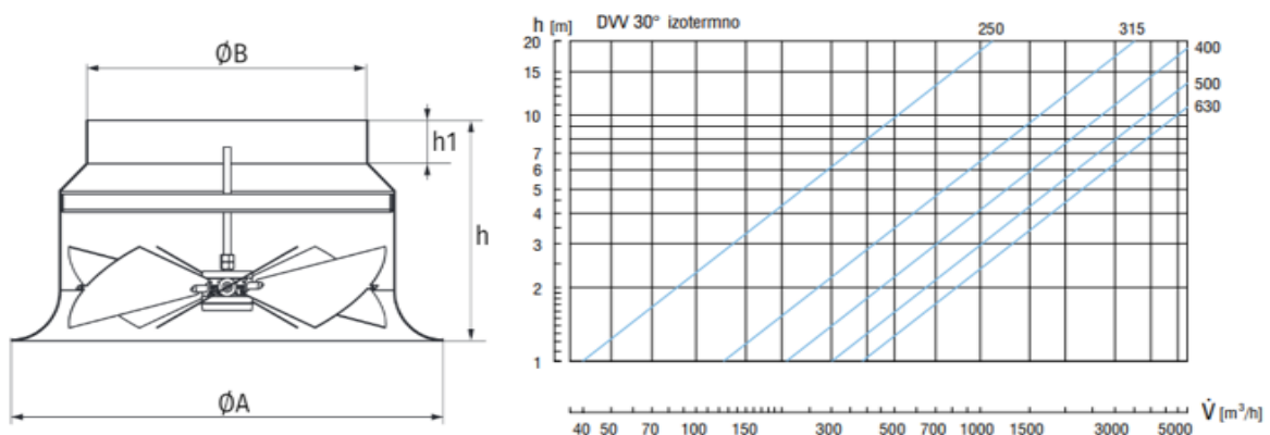
Slika 7.1. Stropni distributer DVV-315 [17]
