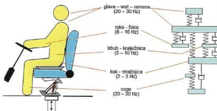
Slika 24. Prijenos vibracija
