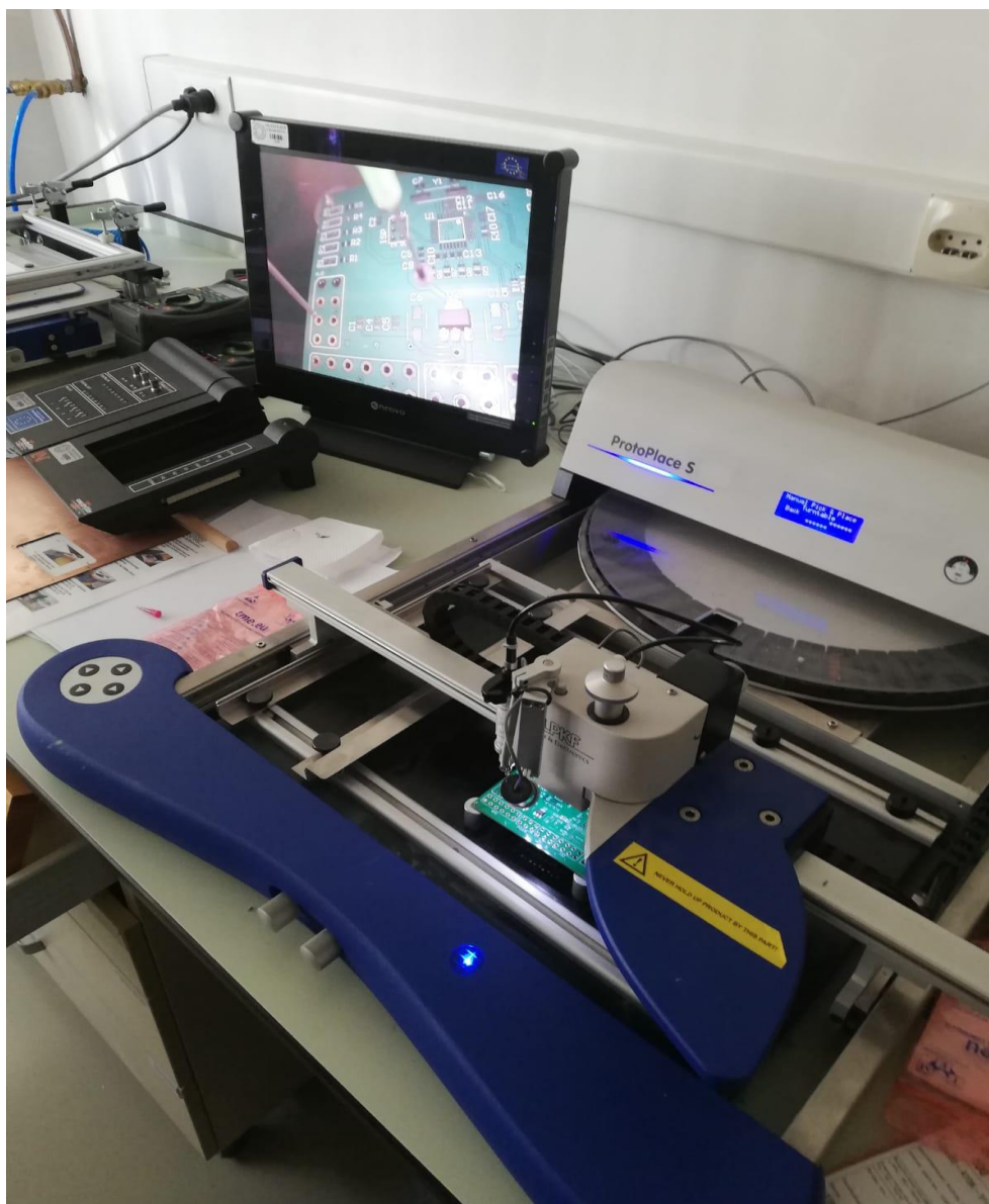
Slika 19: Faza lemljenja
