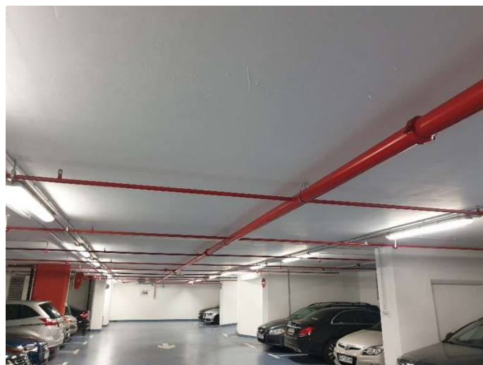
Slika 10. Automatske sprinkler instalacije u garaži HEP-a [13]
