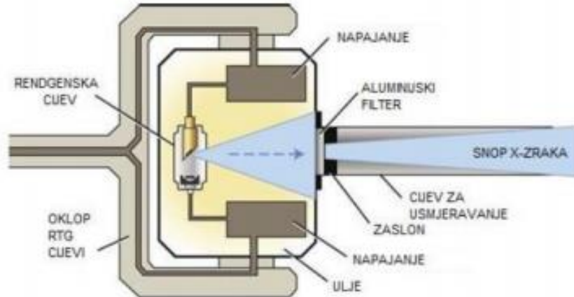
Slika 14. Rendgenska cijev
