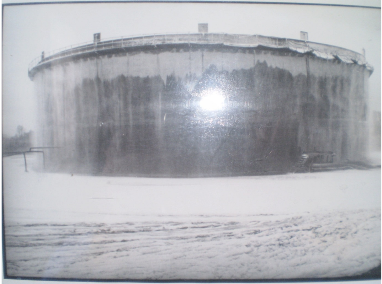
Slika 24. Spremnik R-802 nakon gašenja [7]
