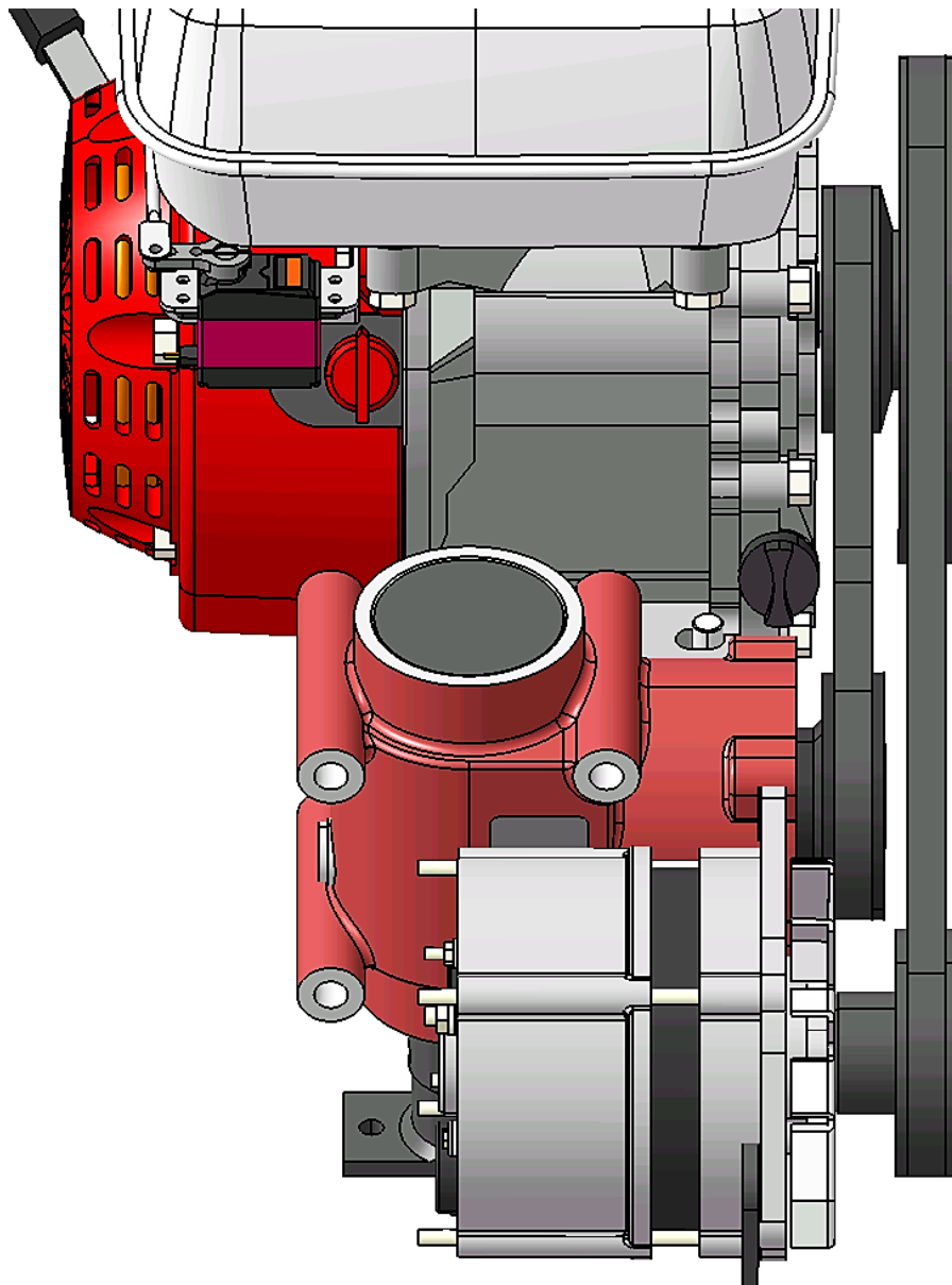
Slika 85 – 3D prikaz modela remenskog sklopa kosilice.
