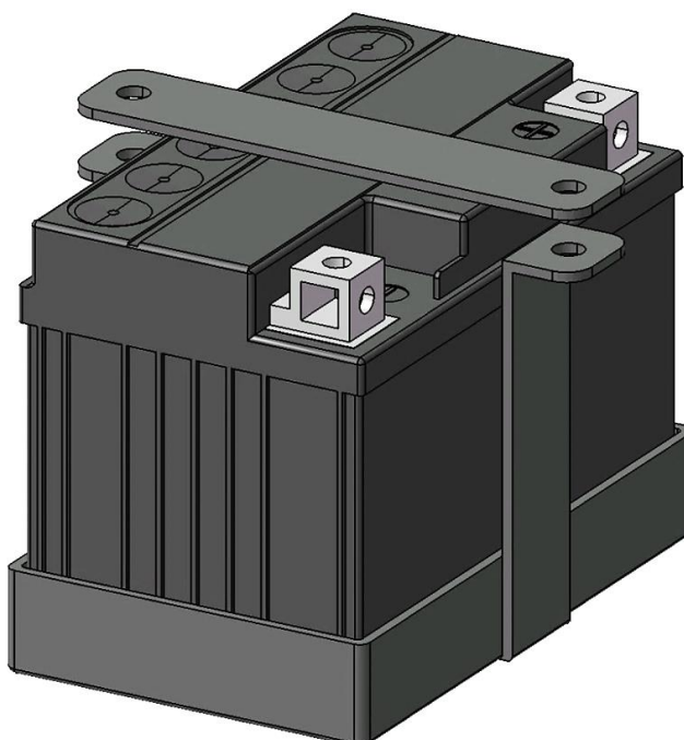
Slika 77 - 3D prikaz modela akumulatora unutar kućišta.
