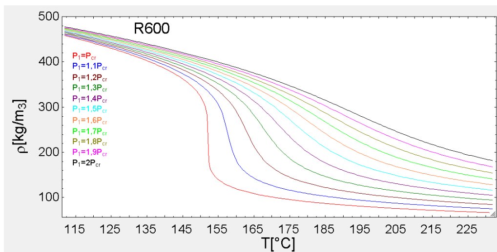
Slika 4-60: Prikaz promjene vrijednosti gustoće u ovisnosti o temperaturi uslijed povećanja vrijednosti nadkritičnog tlaka za radni fluid R600
