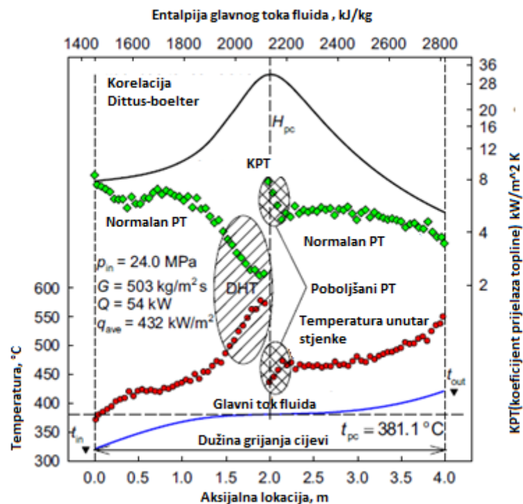
Slika 2-2: Promjena vrijednosti temperature i koeficijenta prijelaza topline duž grijane okomite cijevi kružnog oblika [3](radni fluid je voda, promjer cijevi D=10\text{ mm} , duljina cijevi L= 4\text{ m} .)
