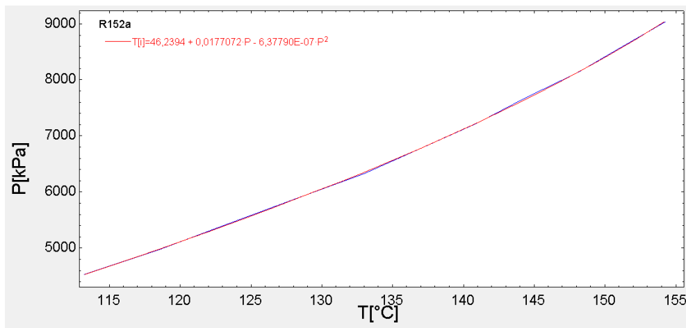
Slika 4-54: Prikaz ovisnosti pseudokritične temperature o nadkričnom tlaku za radni fluid R152a
