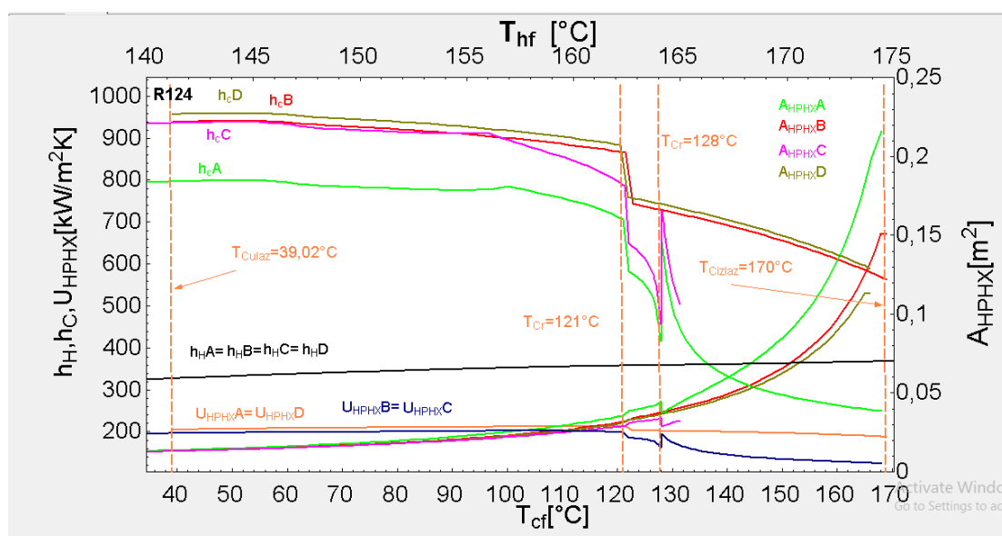
Slika 4-86: Prikaz promjene vrijednosti koeficijenta prijelaza toplote ( h_H , h_C ), ukupnih koeficijenta prolaza toplote ( U_{HPHX} ) i površina segmenata izmjenjivača toplote ( A_{HPHX} ) duž razmatranog izmjenjivača toplote za radni fluid R124
