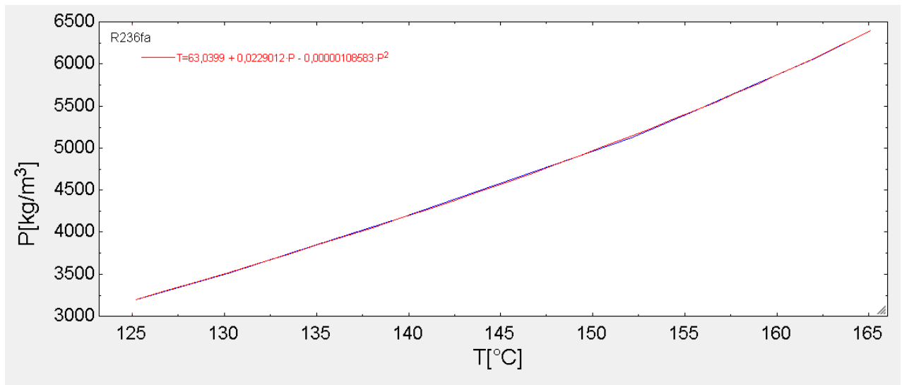
Slika 4-78: Prikaz ovisnosti pseudokrične temperature o nadkričnom tlaku za radni fluid R236fa
