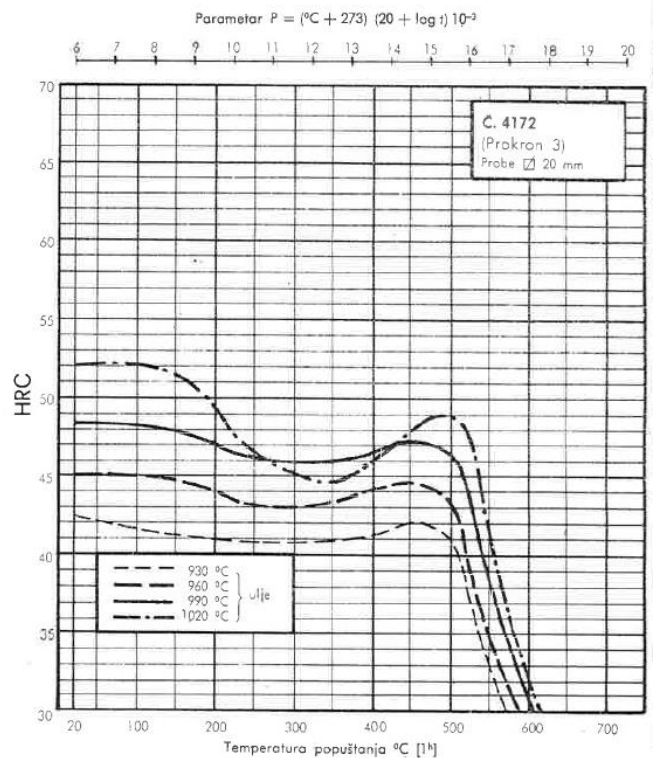
Dijagram popuštanja:
