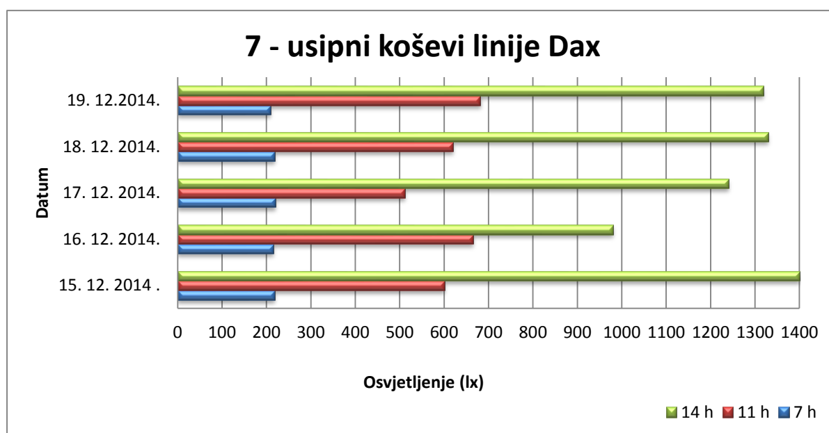
Sl.4.4.2. Grafički prikaz vrijednosti parametara osvjjetljenosti za radno mjesto br. 7
