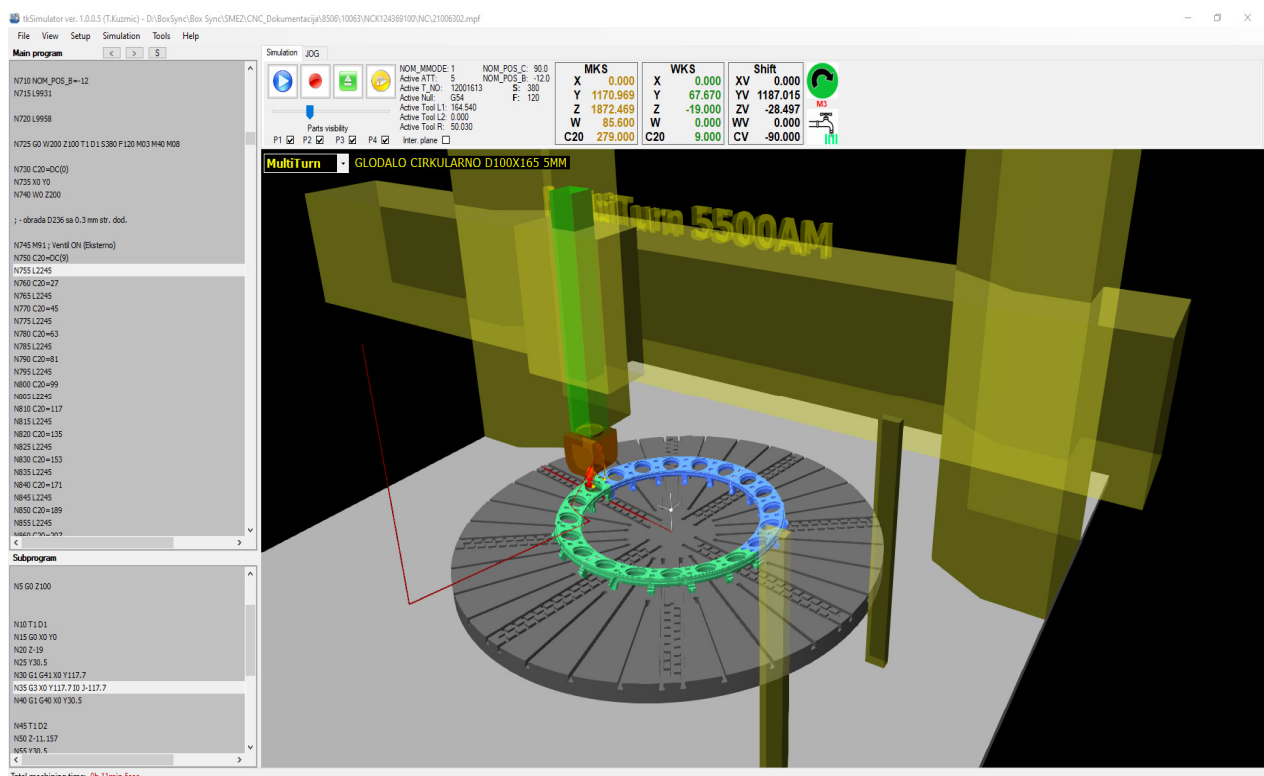
Slika 4.10 Sučelje tkSimulatora [9]
