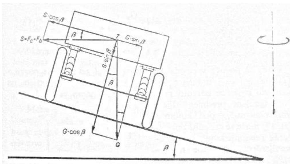
Sl.25. Stabilnost vozila u zavoju [2]
