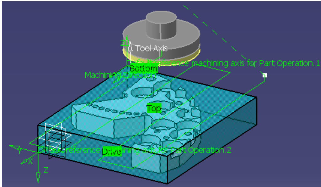
Slika 17. Simulacija putanje alata pri poravnavanju površine
