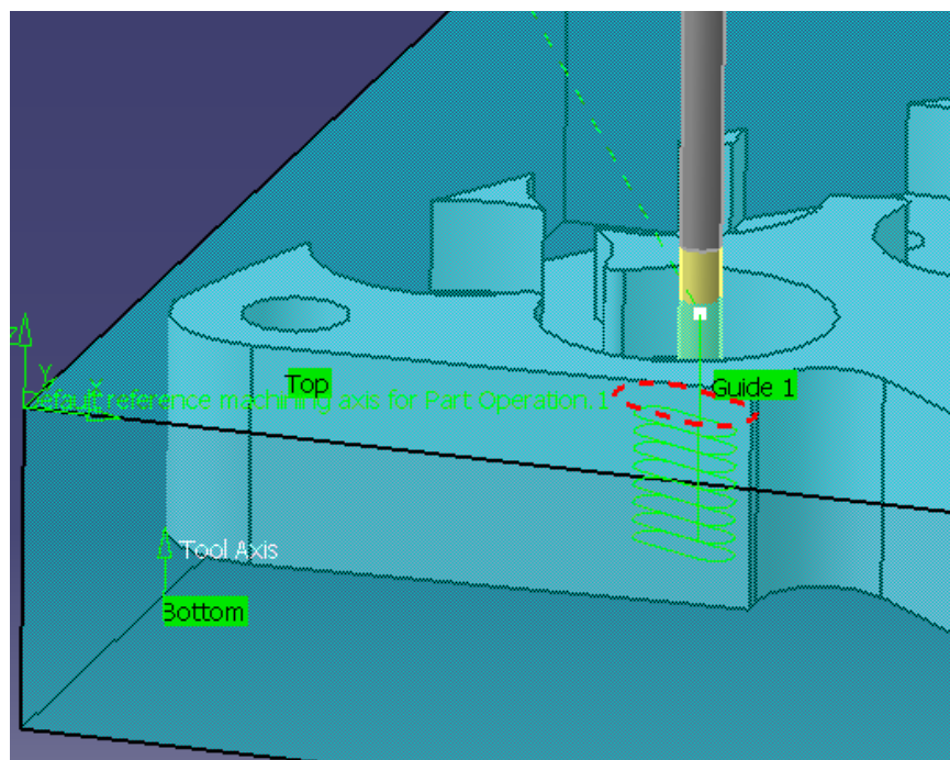
Slika 37. Simulacija putanje petog alata kod obrade četvrtog džepa
