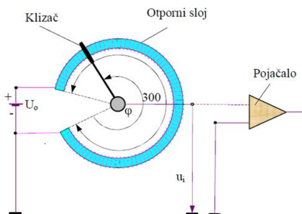
Slika 14. Rotacijski potenciometar
