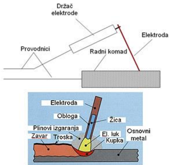
Slika 1-3. Postupak elektrodučnog zavarivanja
