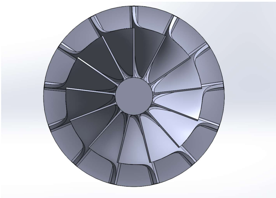
Slika 28: Rotor: pogled 2
