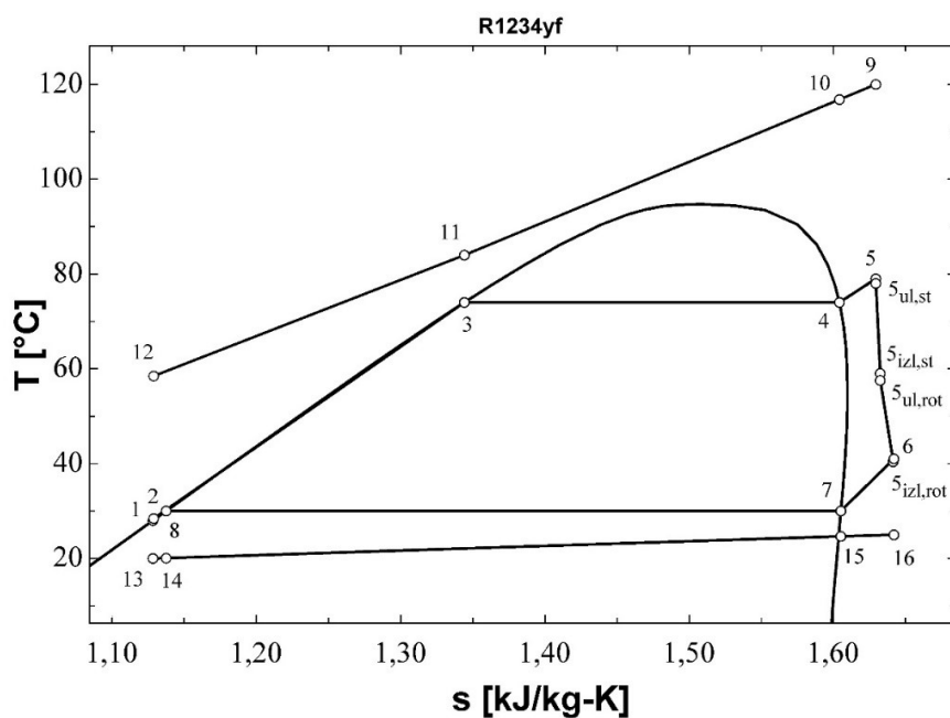
Slika 33: T - s dijagram za rezultate iz tablice 16
