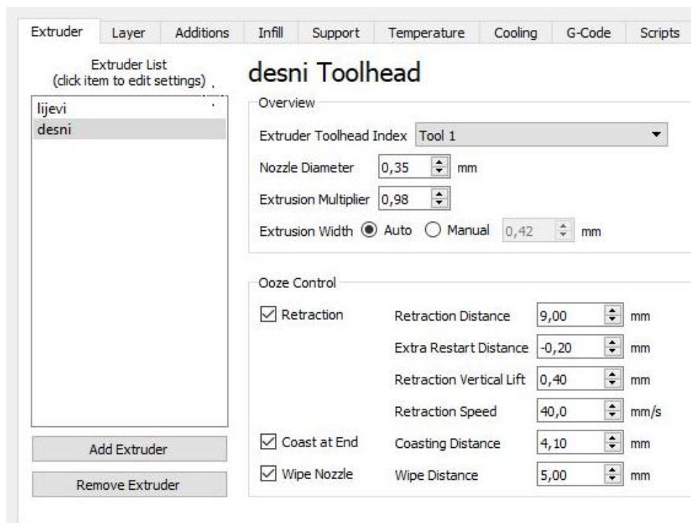
Slika 34. Postavke ekstrudera
