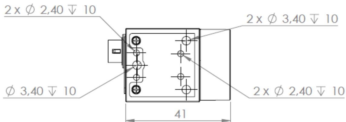
Slika 40. Provrti acA2500-14uc
