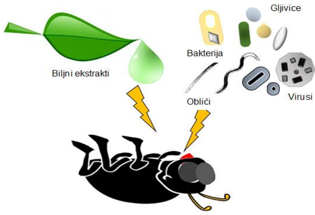
Slika 2. Djelovanje biopesticida [5].
