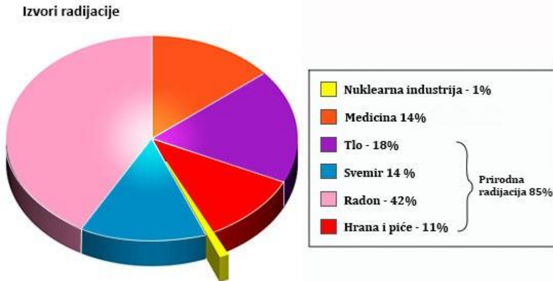
Slika 1. Izvori radijacije
