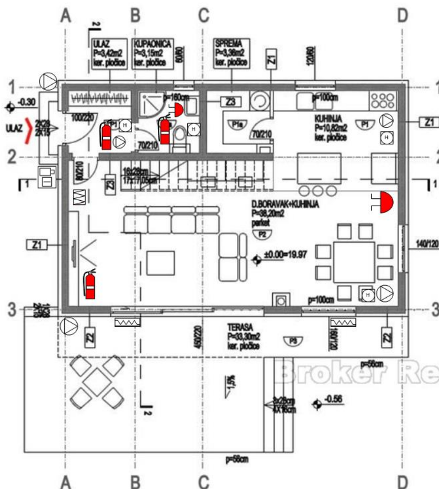
Slika 24. Tlocrt prizemlja s elementima tehničke zaštite
