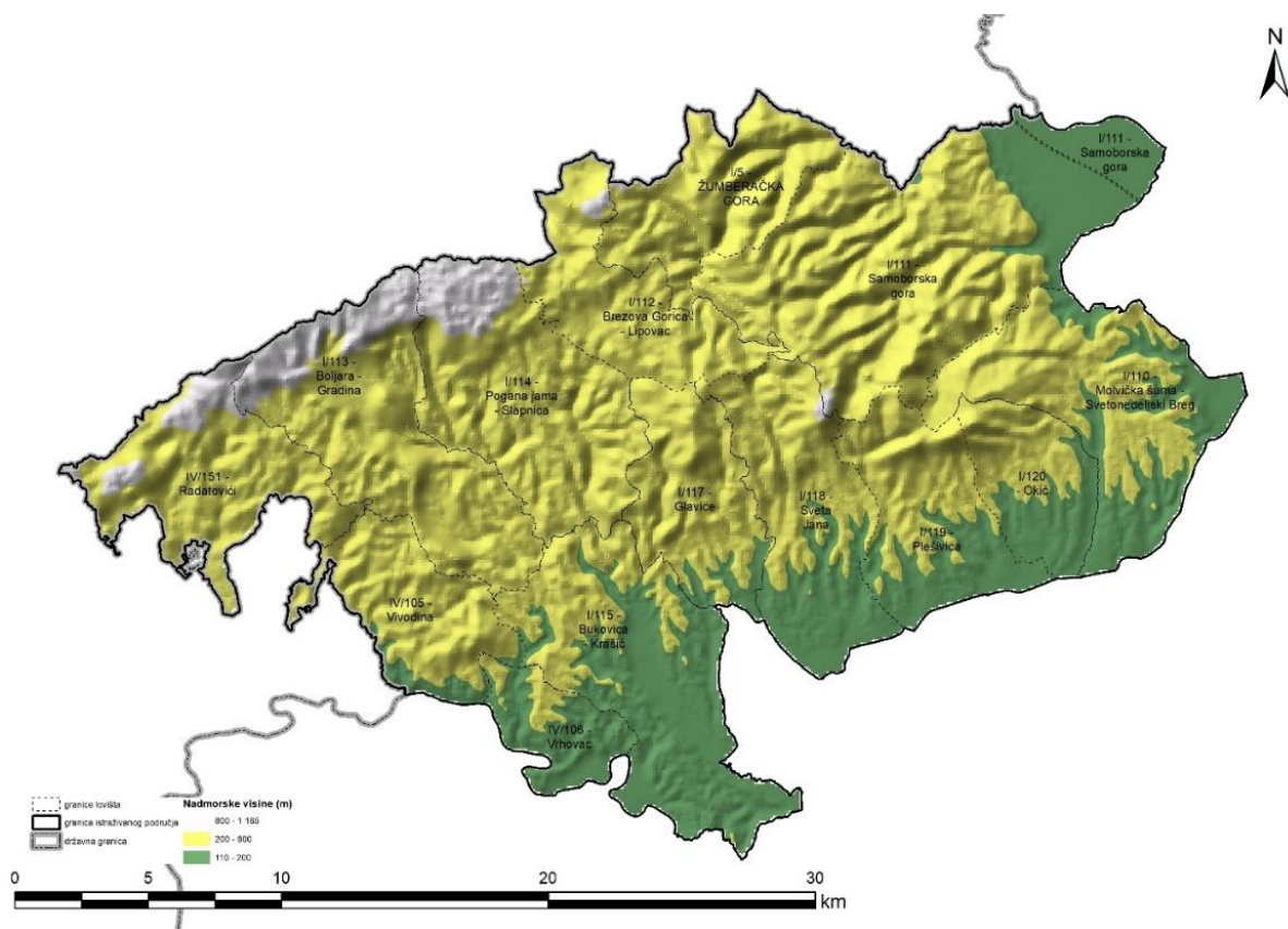
Karta 2. - Prikaz nadmorskih visina za područje Žumberak- Samoborsko gorje (BIŠĆAN, 2020).
