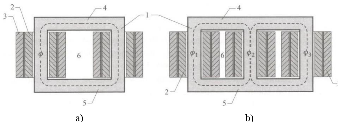
Ilustracija 4. Jezgrasta izvedba transformatora
