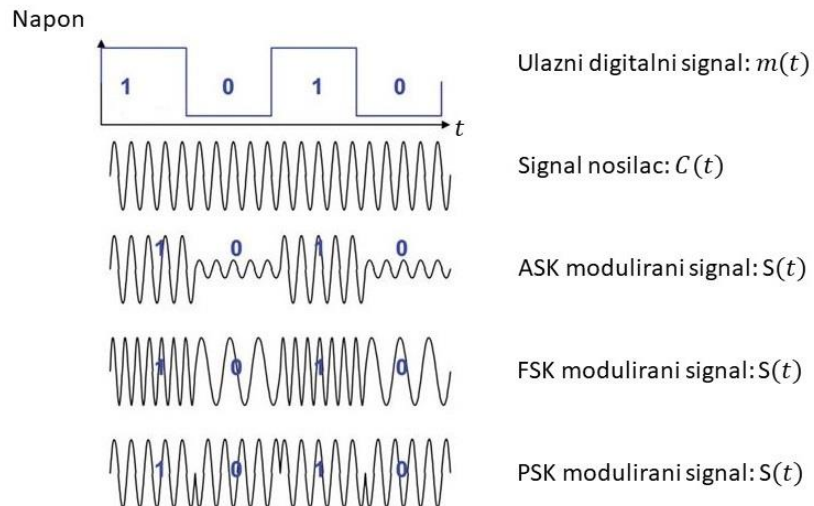
Slika 3. Prikaz digitalno moduliranih signala uz primjenu ASK,FSK i PSK modulacija
