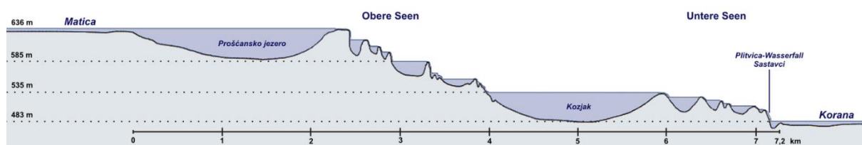
Slika 7: Presjek Plitvičkih jezera
