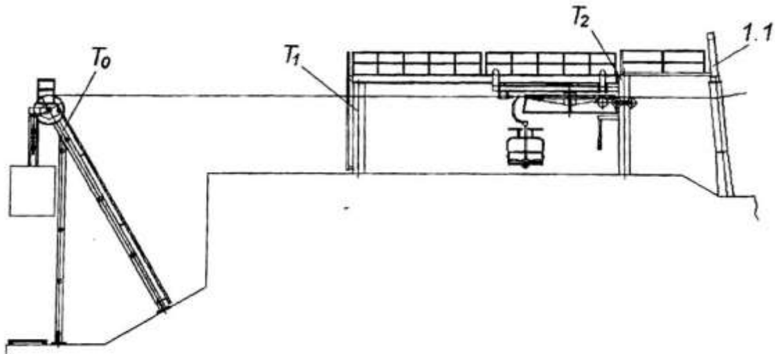
Slika 8 Shematski prikaz donje okretne postaje
